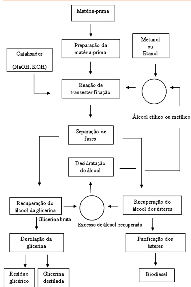
Figura 1: Processo de obtenção do biodiesel
