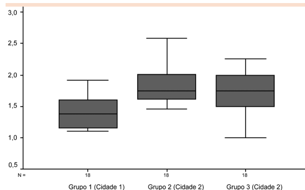
Figura 1: Média da tendência central para os três grupos
