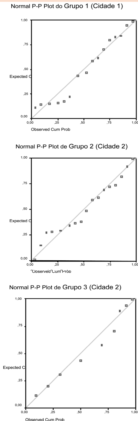
Figura 2: Probabilidade Normal para os três grupos
