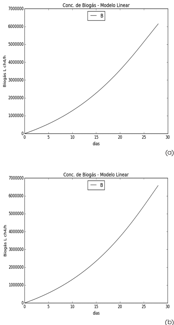
Figura 3: Volume de biogás produzido em Sergipe, por uma indústria com alta DQO, com uma vazão de 2009,2 m 3 de efluente/dia e diferentes concentrações de DQO. (a) 21,3 g O 2 /L e (b) 23,9 g O 2 /L
