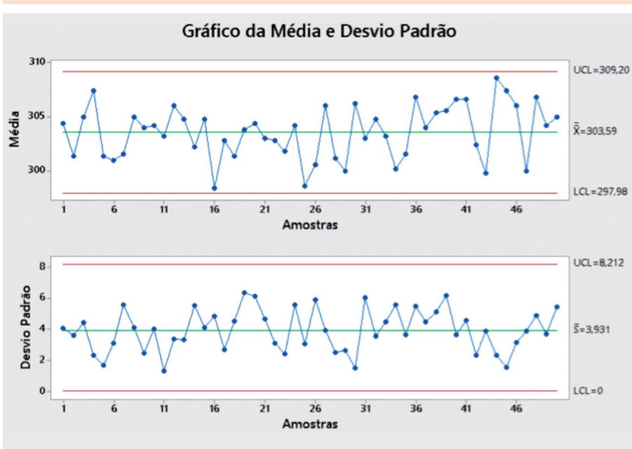
Figura 6: Gráfico da Média e Desvio Padrão (DP)
