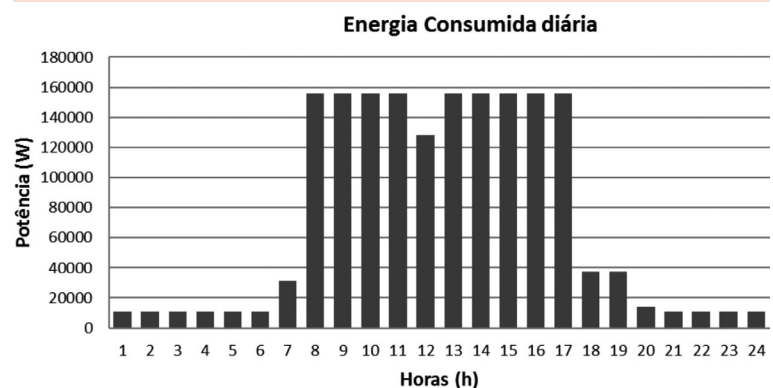
Figura 3: Curva de carga em cada intervalo de hora Fonte: Autores.
