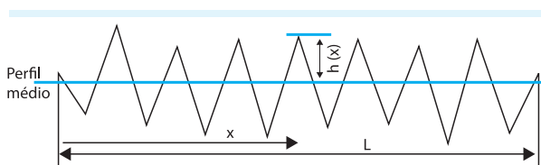
Figura1: Perfil da rugosidade superficial avaliada em Ra
